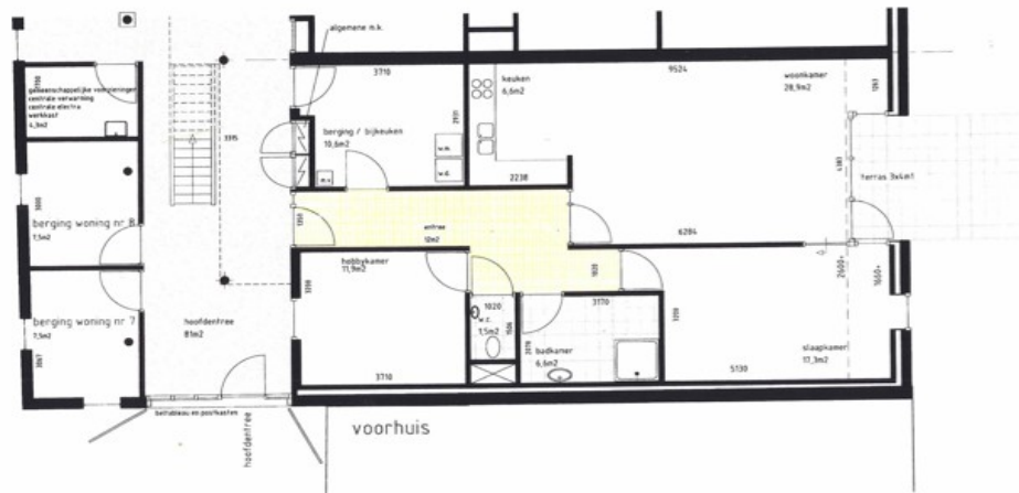
APPARTEMENT NR. 1 begane grond
