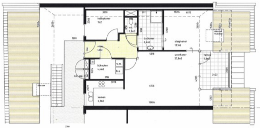
APPARTEMENT NR. 6 1e verdieping
